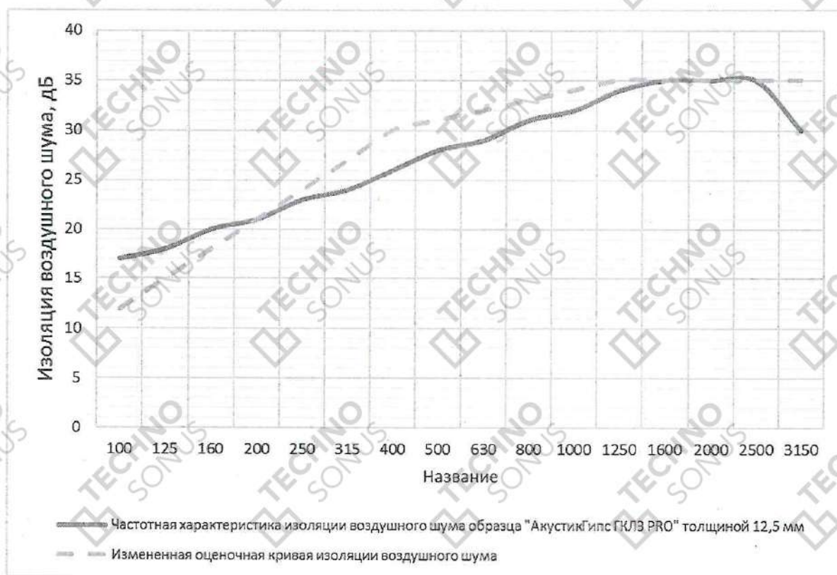
Рисунок 3. График частотной характеристики изоляции воздушного шума образцами «АкустикГипс ГКЛЗ PRO» толщиной 12,5мм
