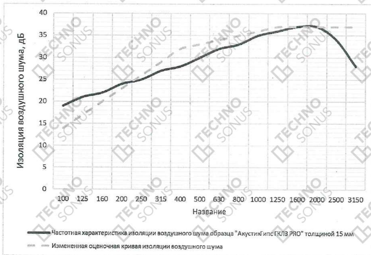
Рисунок 4. График частотной характеристики изоляции воздушного шума образцами звукоизоляционного «АкустикГипс ГКЛЗ PRO» толщиной 15мм
